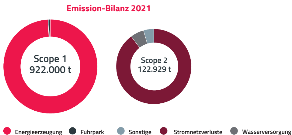
CO 2 -Bilanz 2021 der SachsenEnergie nach Emissionsquelle in t CO 2 -Äquivalente
